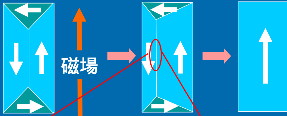
強磁性体の磁化過程
