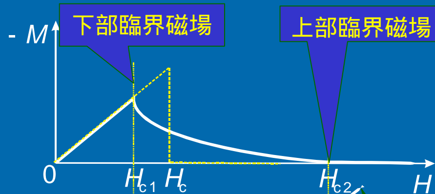
第 種超伝導体
