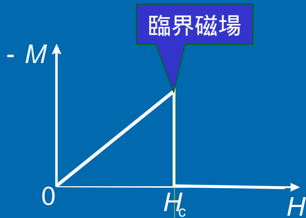
第 種超伝導体
